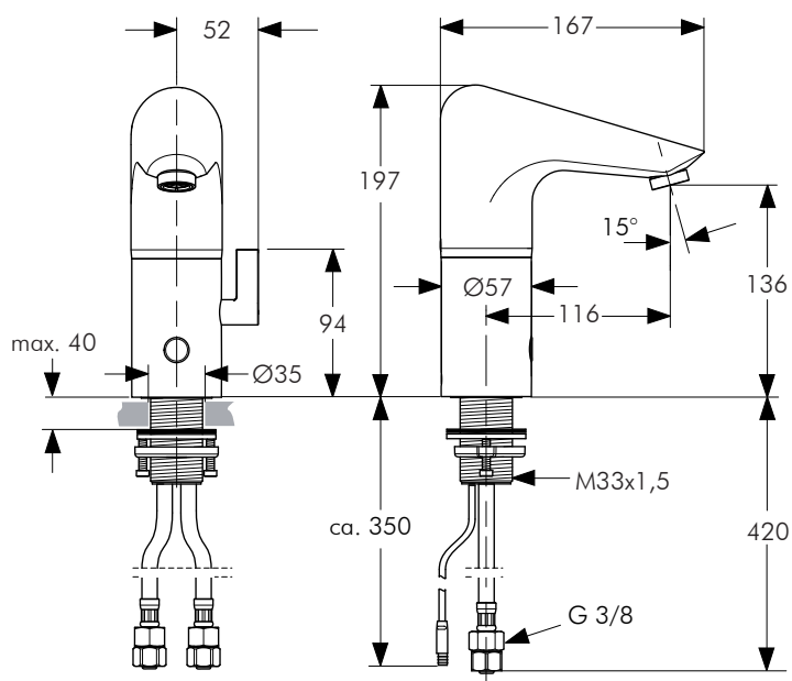
A4152AA med 6V batteri A4154AA med 240V strømforsyning
